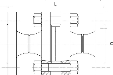
Рис.8. Клапан УРПС БИРС КООФ РН 16,0 МПа
