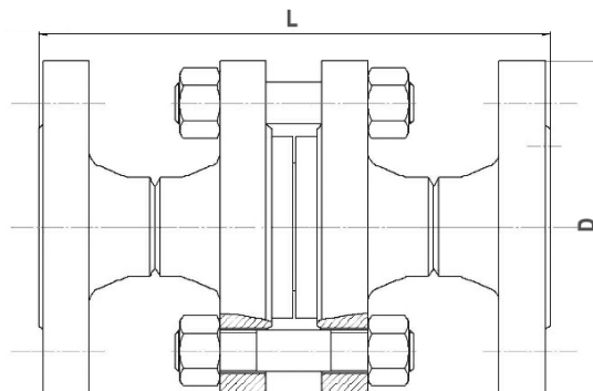
Рис.7. Клапан УРПС БИРС КООФ PN 6,3 МПа
