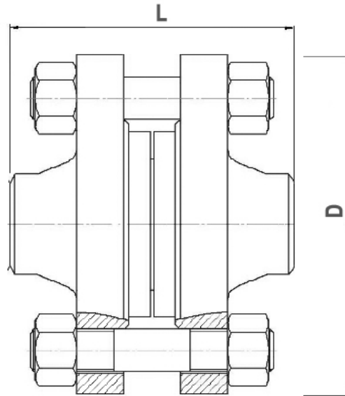
Рис.9. Клапан УРПС БИРС КОО-1 PN 16,0 МПа
