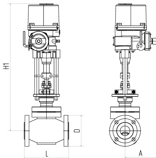
Рис 2 Клапан УРПС БИРС Б01 с электроприводом БИРС 14
