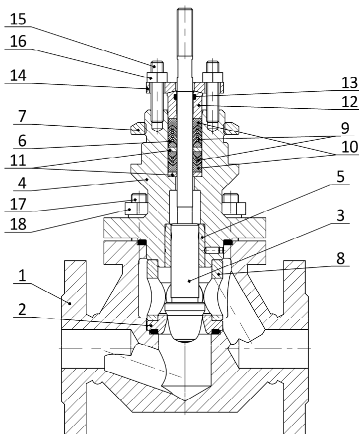
Рисунок 1 – Конструкция клапана
