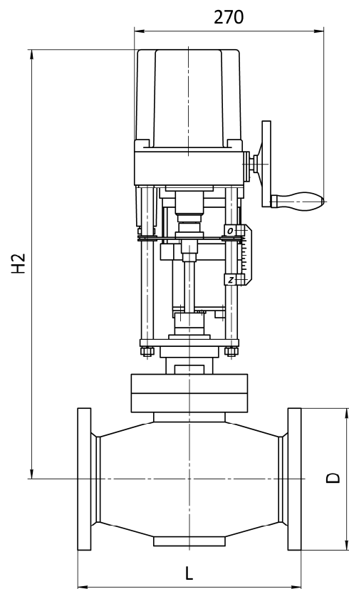
Рис. А.2 – Клапан с электроприводом
