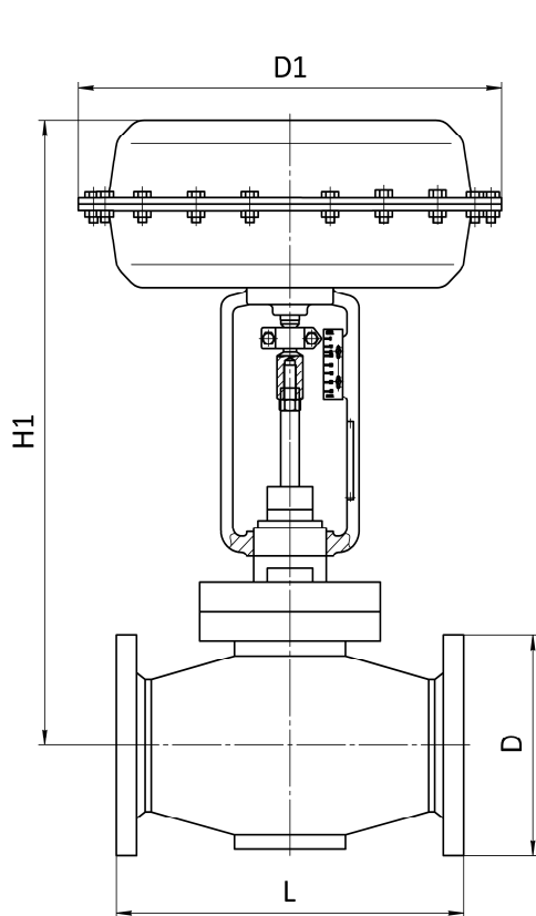
Рис. А.1 – Клапан с МИМ
