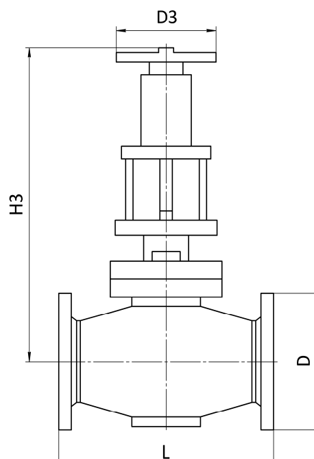
Рис. А.3 – Клапан с ручным приводом
