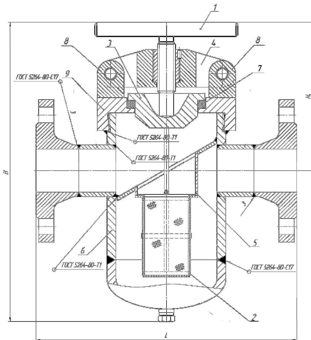
Рисунок. Фильтр сетчатый
